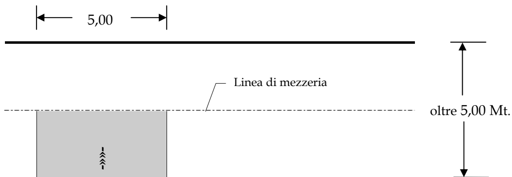
figura 8 scavo trasversale alla carreggiata
